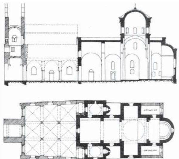
▲ Пресек и основа цркве Светог Спаса
