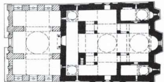
▲ Пресек и основа
