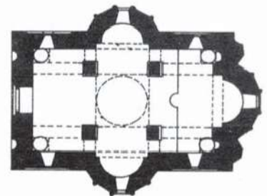
▼ Пресек и основа цркве
